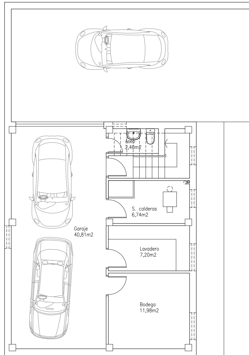
PLANTA SOTANO Sup. Construida 87,97m 2
